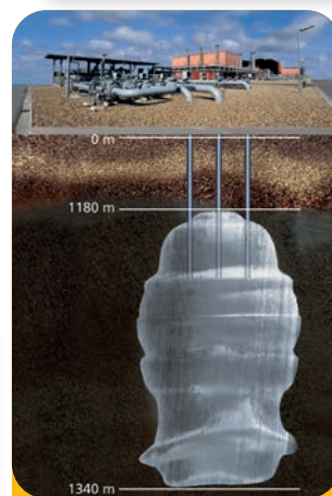
Afb. 4: Schema van een Caverne, Gronau-Epe
